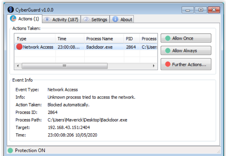
الصورة 1: CyberGuard يكشف و يوقف العمليات الغير موثوقة بطريقة اونوماتيكية
